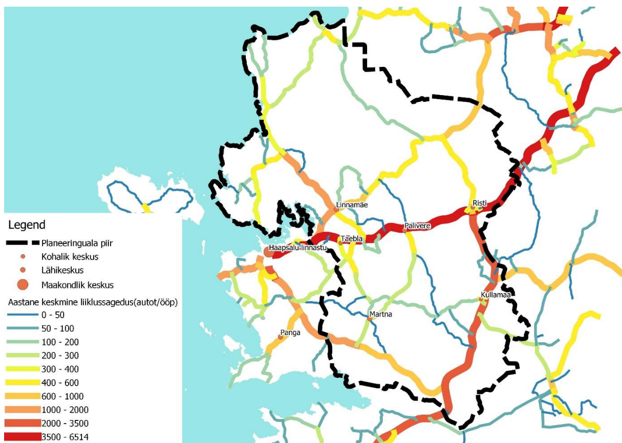
Joonis 3.23. Lääne-Nigula valla riigimaanteede liiklussagedus (Alus: Maa-amet; Maanteeamet, 2020).
